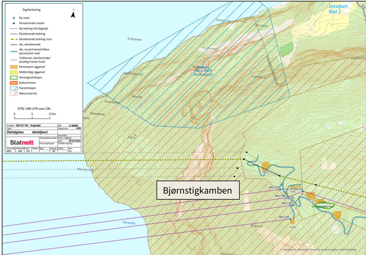
Figur 3: Statnetts detaljplankart av 5. april 2024. Kartet viser permanent riggareal, veier, område for de nye fjordspennbukkene, ny trasé for ledningen og eksisterende ledning på Bjørnstigkamben.
