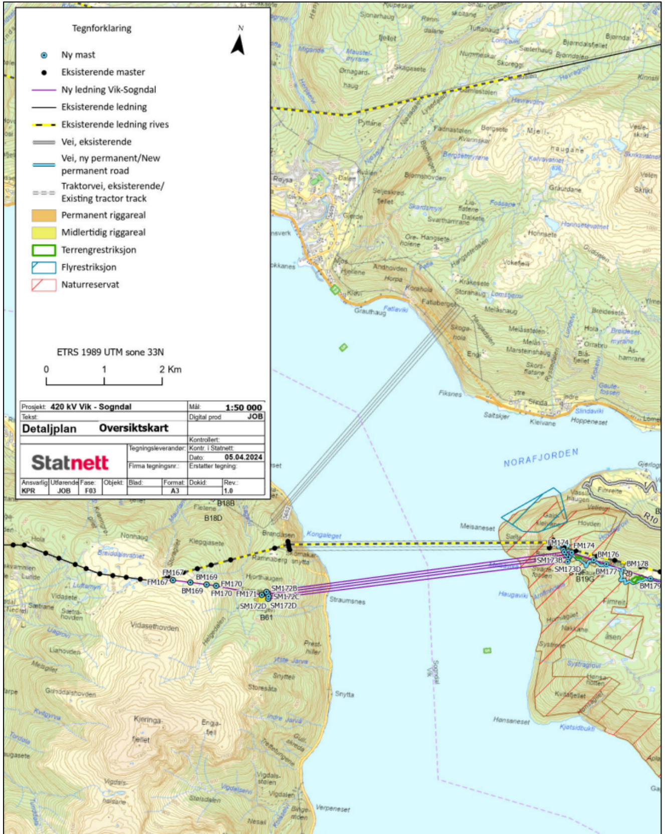
Figur 1: Utsnitt av Statnetts oversiktskart av 5. april 2024. Eksisterende fjordspenn som skal rives vises med gul og sort stiplede linje, mens nytt vises med lilla linjer.
