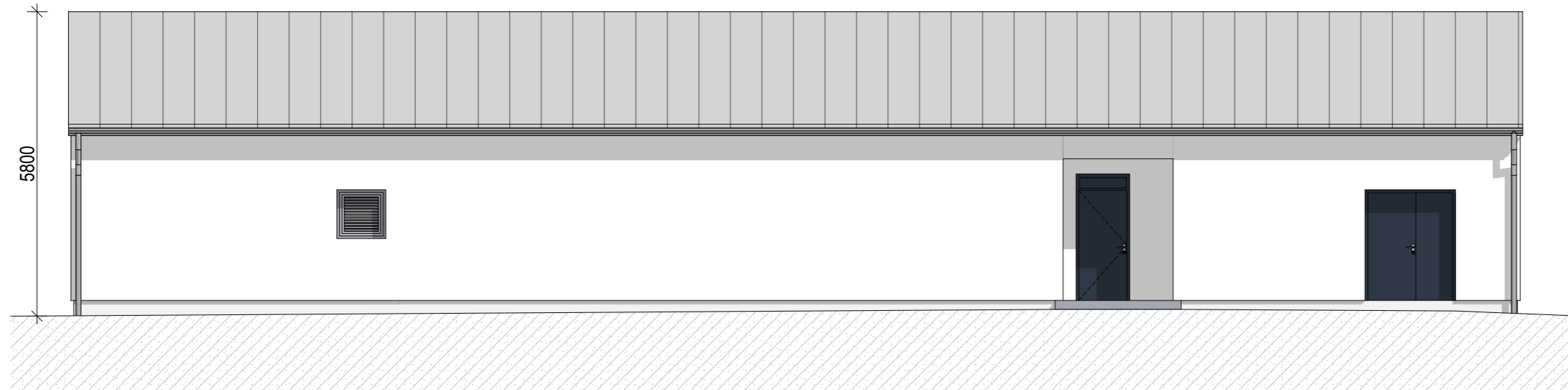
1:100 Fasade Nord Vest
