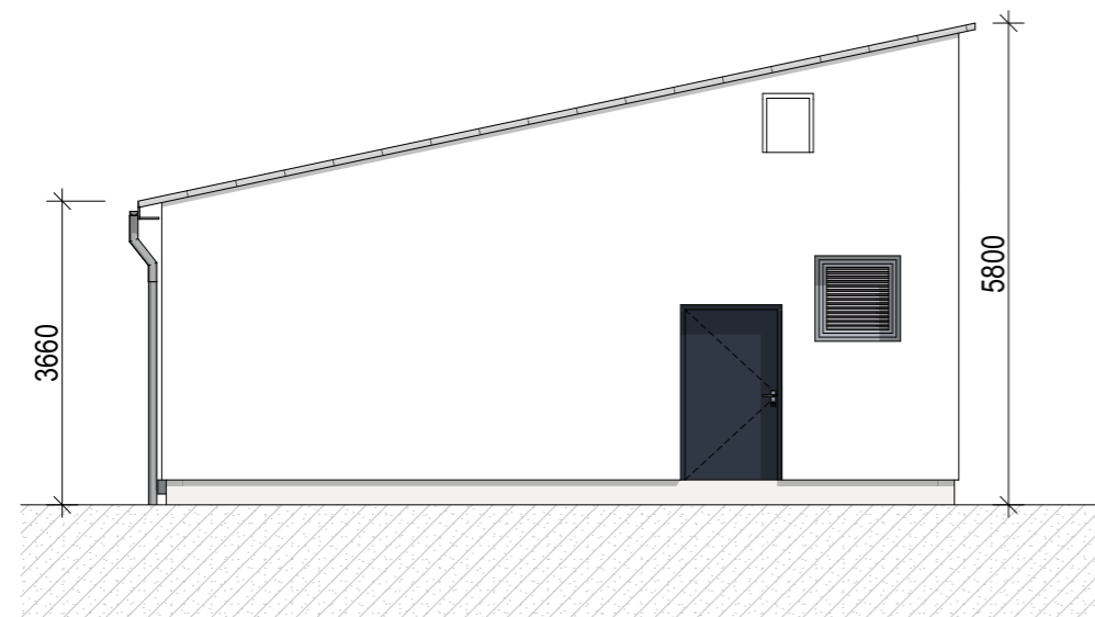
1:100 Fasade Sør Vest
