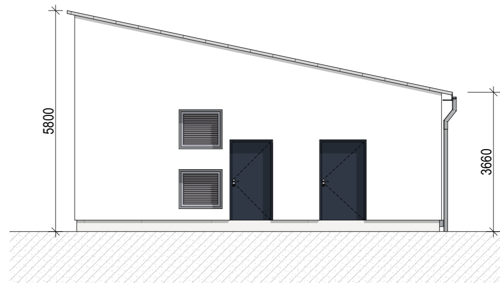
1:100 Fasade Nord Øst
