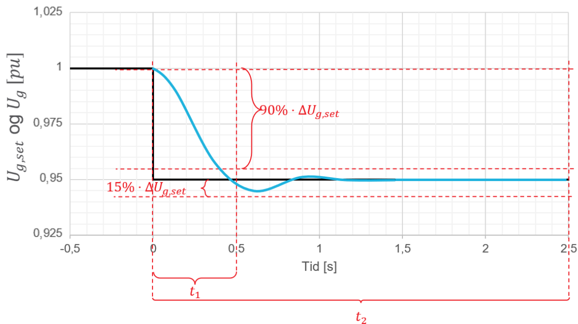
FIGUR 13-16: ILLUSTRASJON AV KRAV TIL UTREGULERINGSTID AV SPENNINGREFERANSESTEG I NEGATIV RETNING FOR MAGNETISERINGSUTSTYR I LUKKET SLØYFE MED ÅPEN EFFEKTBRUYTER FOR SYNKRONE PRODUKSJONSENHETER.
