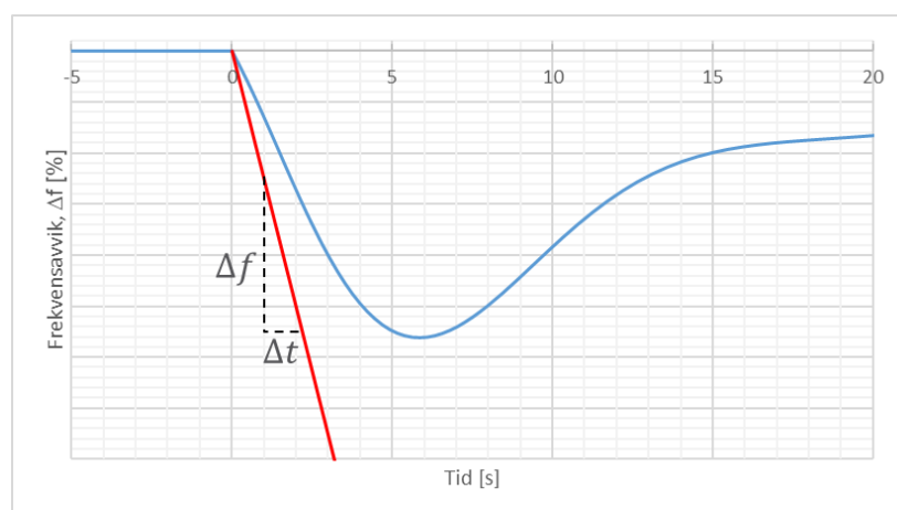
FIGUR 14-2: ILLUSTRASJON AV KRAV TIL FREKVENSDRINGSHASTIGHET. DERSOM FREKVENSFØRSLØPET ER OVER DEN RØDE LINJEN, SOM FALLER MED EN FREKVENSDRINGSHASTIGHET PÅ \frac{\Delta f}{\Delta t} = 1,5 Hz/s , SKAL PRODUKSJONSENHETEN OPERERE NORMALT.
