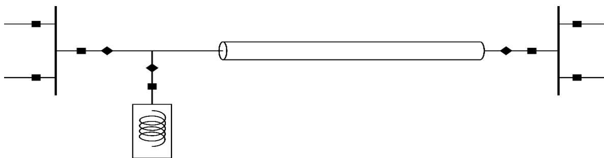
FIGUR 5-5: EKSEMPEL PÅ T-AVGRENING MED BRYTER TIL KOMPENSERINGSANLEGG - BEHOVSPRØVD FLEKSIBILITET I FORHOLD TIL AT KOMPENSERINGSANLEGGET IKKE KAN VÆRE TIL NYTTE FOR KRAFTSYSTEMET NÅR SJØKABEL IKKE ER I DRIFT
