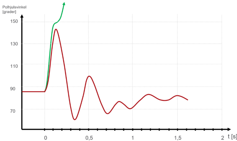
FIGUR 13-4: TYPISK TIDSFORLØP FOR ROTORVINKEL I TILKNYTNINGSPUNKT NÅR SYNKRONISME MOT NETTET BEHOLDES (RØD) OG TAPES (GRØNN).
