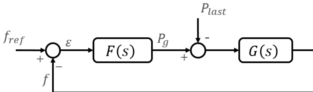
FIGUR 13-12: LUKKET SLØYFE
