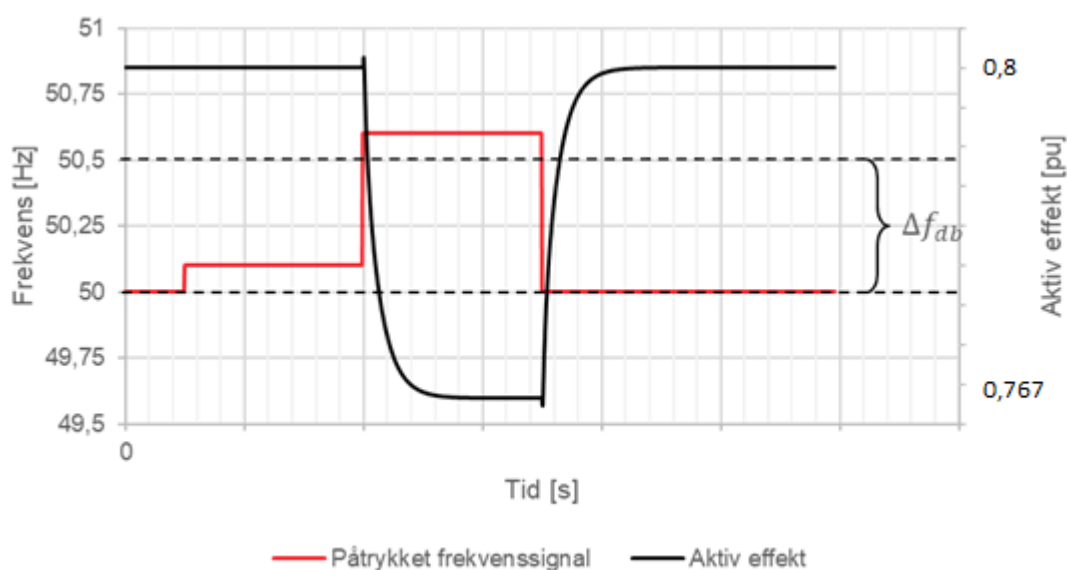
FIGUR 19-4 ILLUSTRASJON AV PRØVE FOR AKTIV EFFEKTRRESPONS (SORT) VED PÅTRYKKET FREKVENNSTEG(RØD) MED AKTIVE DØDBÅND (SORT STIPILET LINJE).
