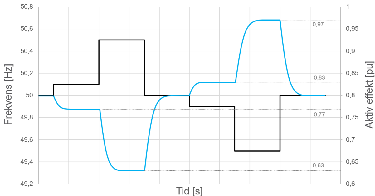
FIGUR 13-25: TEST AV EFFEKTPRESPONS (BLÅ) VED PÅTRYKKET FREKVENSSPRANG (SORT).
