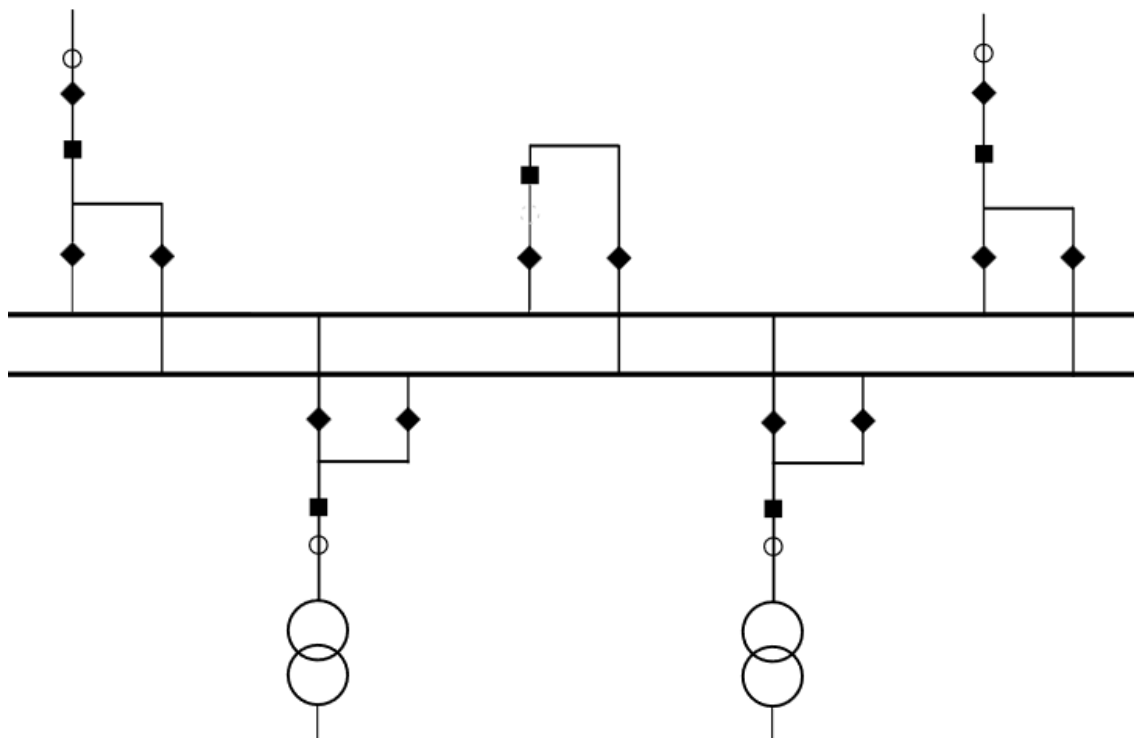
FIGUR 5-3: EKSEMPEL PÅ STASJONSLØSNING MED FLEKSIBILITET FOR REGIONALE KOBLINGSANLEGG MED NOMINELL SYSTEMSPENNING 110 \leq U_n < 220 kV; AB SAMLESKINNE, ENKLE EFFEKTBRYTTERE, ENKLE STRØMTRANSFORMATORER OG DOBLE SKILLEBRYTTERE, SAMT SAMMENKOBLINGSFELT.
