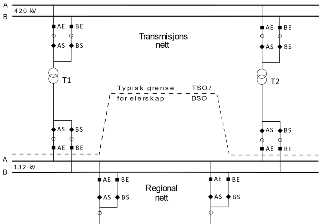
FIGUR 5-3: ALTERNATIVT EKSEMPEL PÅ KOBLINGSANLEGG FOR REGIONALNETTSTASJON TILKNYTTET TRANSMISJONSNETT: LUFTISOLERT ANLEGG MED AB SAMLESKINNE, DOBLE EFFEKTBRYTERE, SKILLEBRYTERE OG ENKLE STRØMTRANSFORMATORER, MEN DOBLE STRØMTRANSFORMATOR PÅ AVGANGER TIL TRANSMISJONSNETT I STEDET FOR SAMMENKOBLINGSBRYTER.
