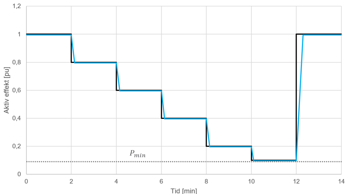
FIGUR 16-4: AKTIV EFFEKTRESPONS (BLÅ) VED PÅTRYKKET SETTPUNKT (SORT).
