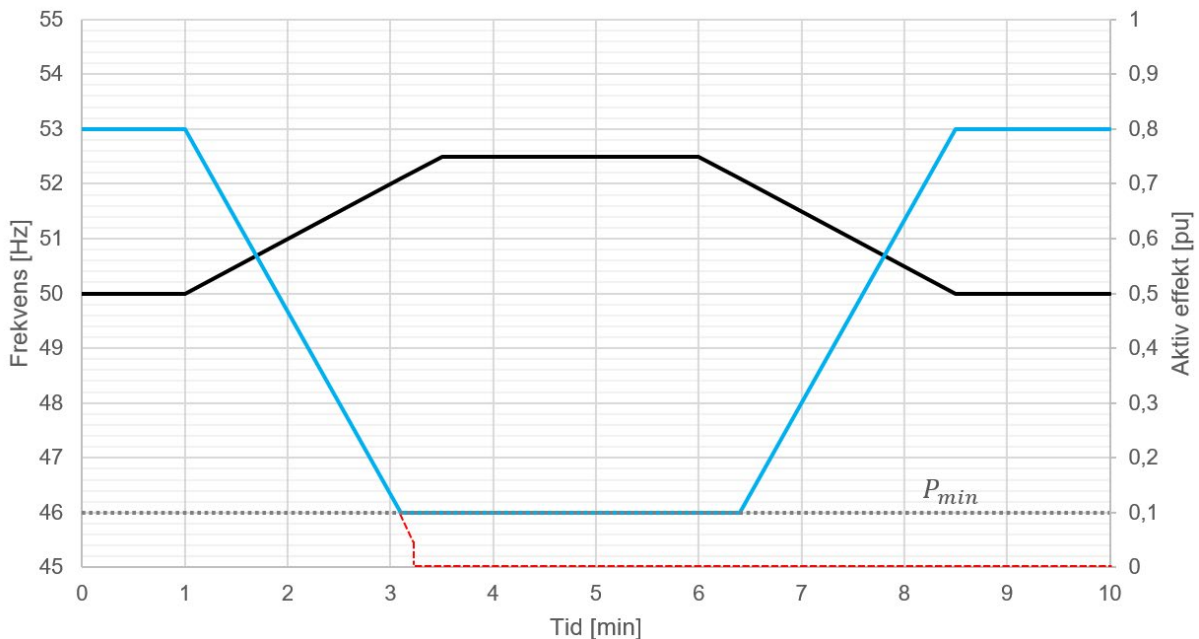
FIGUR 16-9: AKTIV EFFEKTRESPONS (BLÅ) VED PÅTRYKKET FREKVENSRAMPE (SORT). VED 52,5 Hz HOLDER PARKEN SETTPUNKTET P_{min} ISTEDEFOR Å KOBLE UT ELLER GÅ TIL STOPP (RØD STIPLET LINJE).
