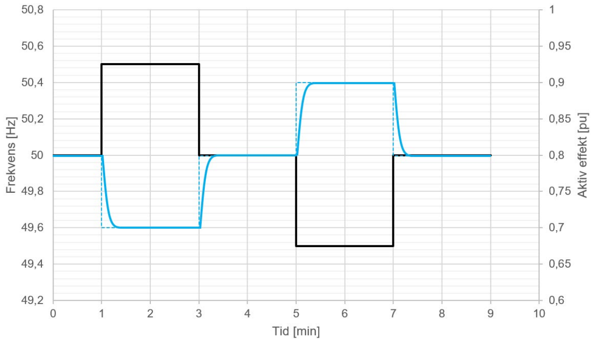
FIGUR 16-8: AKTIV EFFEKTRESPONS (BLÅ) VED PÅTRYKKE FREKVENSSPRANG (SORT) UTEN DØDBÅND MED STATIKK PÅ 10%.
