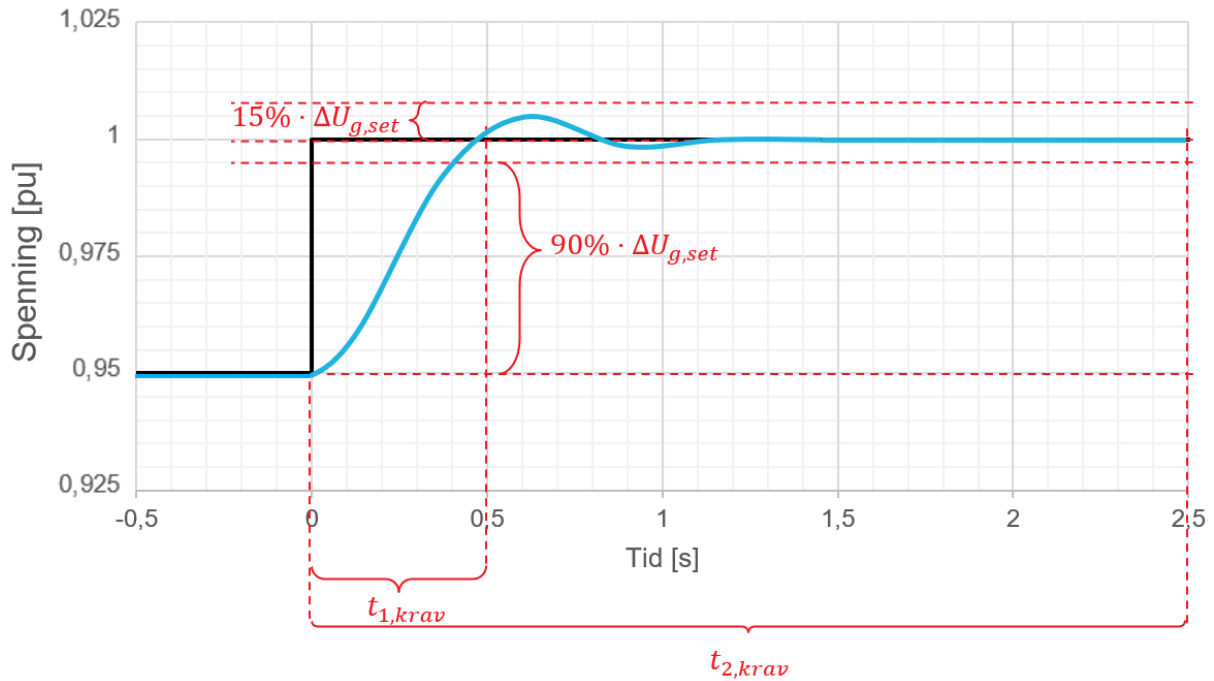
FIGUR 13-34: ILLUSTRASJON AV UTREGULERINGSTID I NEGATIV RETNING FOR MAGNETISERINGSUTSTYR.
