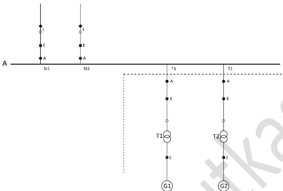
FIGUR 5-4 FIGUR 5-5: EKSEMPEL PÅ STASJONSANLEGG MED ENKEL FLEKSIBILITET
