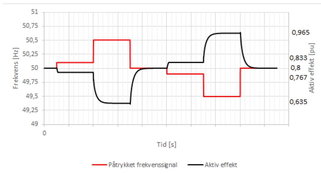
FIGUR 19-3: ILLUSTRASJON AV PRØVE FOR AKTIV EFFEKTRESPONS (SORT) VED PÅTRYKKET FREKVENNSTEG (RØD)
