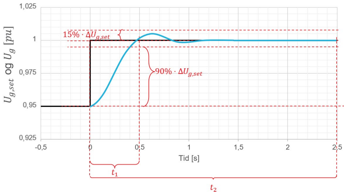
FIGUR 12-8: ILLUSTRASJON AV KRAV TIL UTREGULERINGSTID AV SPENNINGSETTPUNKT I POSITIV RETNING FOR MAGNETISERINGSUTSTYR I LUKKET SLØYFE MED ÅPEN EFFEKTBYTER FOR SYNKRONE PRODUKSJONSENHETER.
