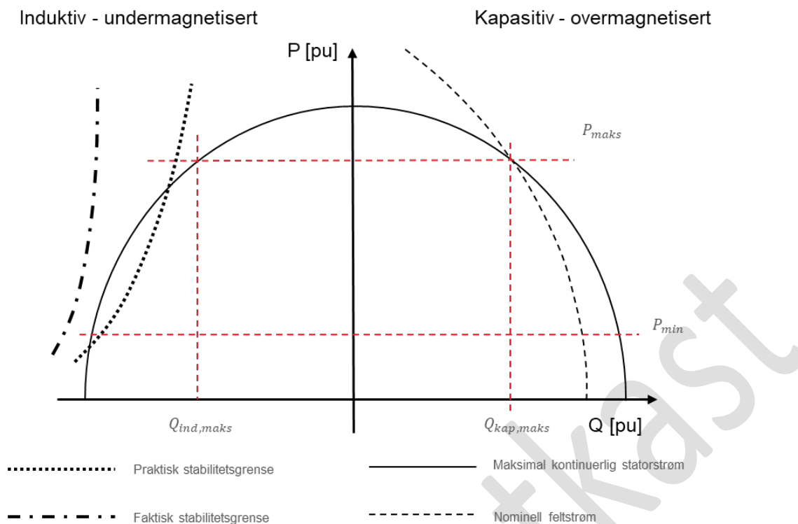
FIGUR 12-7: DRIFTSDIAGRAMMET TIL EN TYPISK SYNKROGENERATOR
