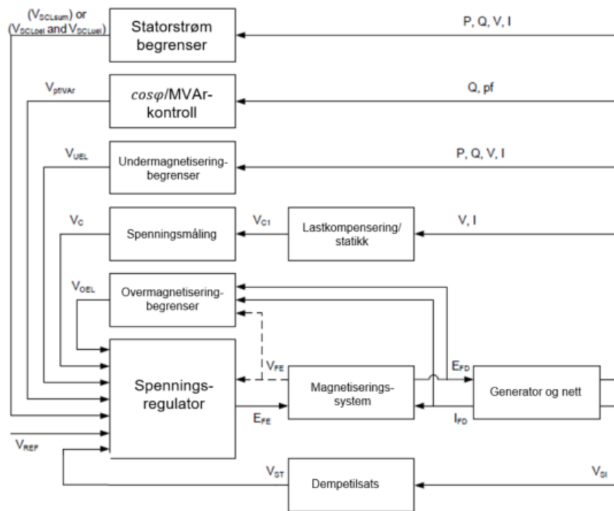
FIGUR 13-14: PRINSIPIELL VIRKEMÅTE TIL SPENNINGREGULATOREN FOR EN SYNKRON PRODUKSJONSENHET [11]. NB; MERK AT BLOKKDIAGRAMMET KUN VISER SPENNINGINNANG TIL DEMPETILSATS. DEMPETILSATS SKAL OGSÅ BENYTTE TURTALL IHT. KRAV I KAPITTEL 12.5.6.
