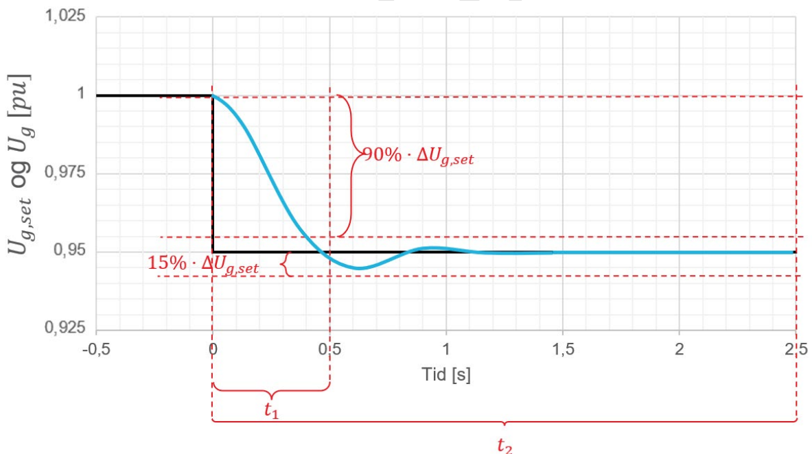
FIGUR 12-9: ILLUSTRASJON AV KRAV TIL UTREGULERINGSTID VED SPRANG SPENNINGSETTPUNKT I NEGATIV RETNING FOR MAGNETISERINGSUTSTYR I LUKKET SLØYFE MED ÅPEN EFFEKTBYTER FOR SYNKRONE PRODUKSJONSENHETER.
