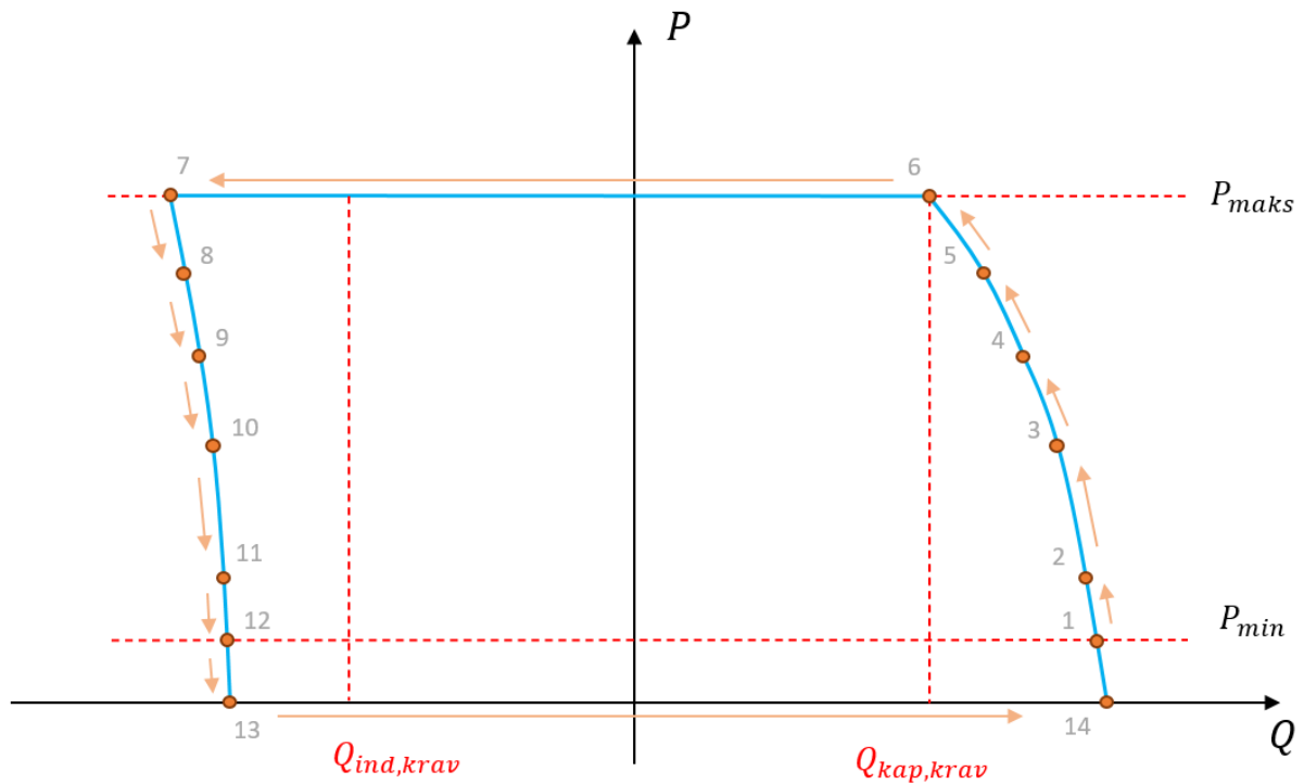
FIGUR 16-15: ILLUSTRASJON AV PROSEDYRE FOR DOKUMENTASJON AV REAKTIV YTELSE FOR EN KRAFTPARK, HER MED STATCOM-FUNKSJONALITET OG UTEN REGULERBART KONDENSATORBATTERI. ORANSJE PUNKTER MÅRKERER MÅLEPUNKTER SOM DOKUMENTERES.
