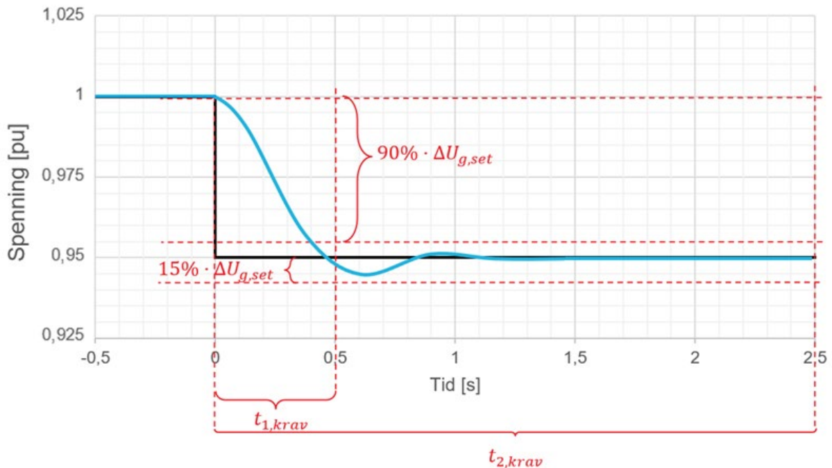
FIGUR 13-33: ILLUSTRASJON AV UTREGULERINGSTID I NEGATIV RETNING FOR MAGNETISERINGSUTSTYR.
