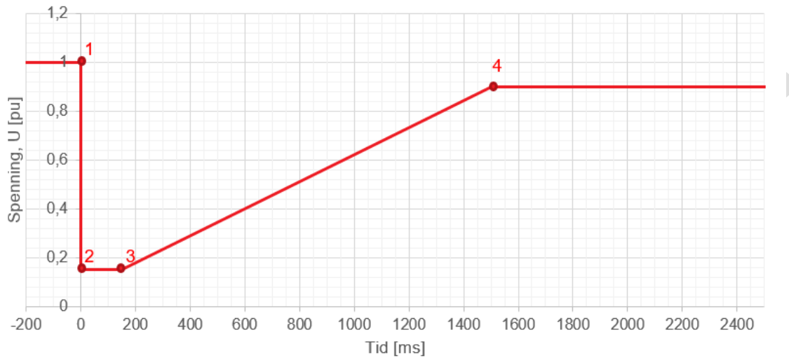
FIGUR 14-10: KRAV TIL FAULT RIDE THROUGH FOR KRAFTPARKER AV TYPE A, B OG C, OG TYPE D TILKNYTTET SPENNINGSNIVÅ < 110 kV. KRAFTPARKEN SKAL VÆRE TRANSIENT STABIL OG OPPRETTHOLDE PRODUKSJONEN FOR ALLE FEILFORLØP SOM GIR EN SPENNING I TILKNYTNINGSPUNKTET OVER KURVEN.
