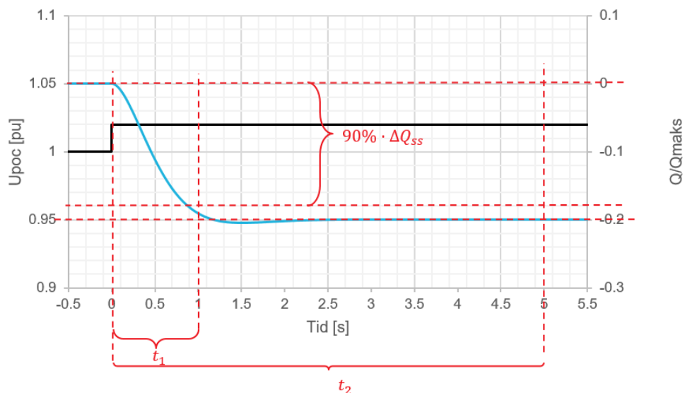
FIGUR 14-6: REAKTIV EFFEKTRESPONS VED STEGVIS ENDRING I SPENNING PÅ HHV \pm 2\% . KRAV ER MARKERT I RØDSTIPLEDE LINJER.
