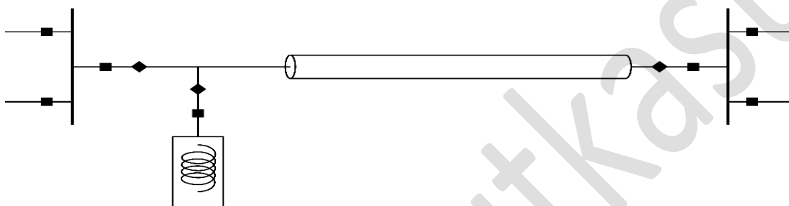
FIGUR 5-5 FIGUR 5-6: EKSEMPEL PÅ T-AVGRENING MED BRYTER TIL KOMPENSERINGSANLEGG - BEHOVSPRØVD FLEKSIBILITET I FORHOLD TIL AT KOMPENSERINGSANLEGGET IKKE KAN VÆRE TIL NYTTE FOR KRAFTSYSTEMET NÅR SJØKABEL IKKE ER I DRIFT
