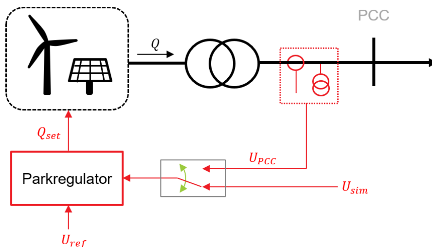
FIGUR 16-13: FORENKLET ILLUSTRASJON AV SPENNINGREGULERING VED EKSTERNT SIMULERT SIGNAL FOR NETTSPENNING UTEN TILBAKEKOBLING AV MÅLT NETTSPENNING.
