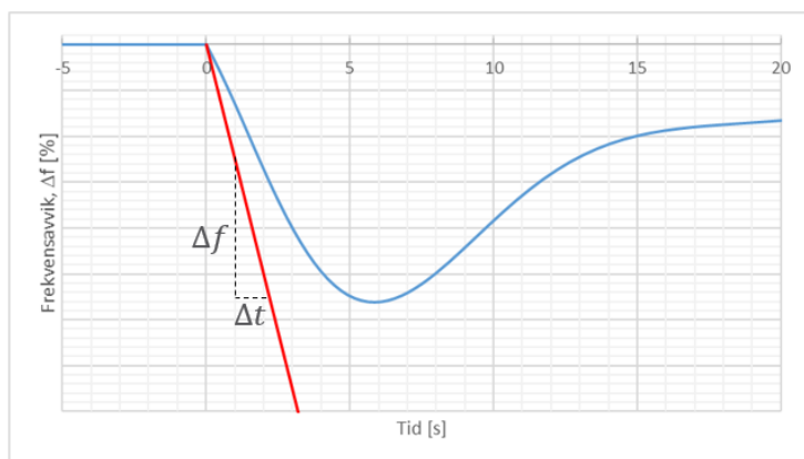
FIGUR 12-3: ILLUSTRASJON AV KRAV TIL FREKVENSDRINGSFASTHET. DERSOM FREKVENSFORLØPET ER OVER DEN RØDE LINJEN, SOM FALLER MED EN FREKVENSDRINGSFASTHET \frac{\Delta f}{\Delta t} = 1,5 \text{ Hz/s} , SKAL PRODUKSJONSENHETEN OPERERE NORMALT.
