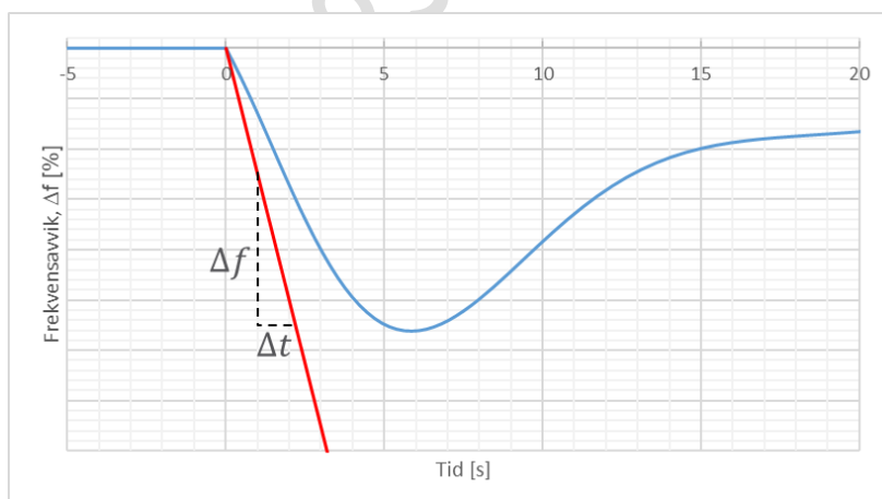
FIGUR 14-2: ILLUSTRASJON AV KRAV TIL FREKVENSEDRINGSHASTIGHET. DERSOM FREKVENSFORLØPET ER OVER DEN RØDE LINJEN, SOM FALLER MED EN FREKVENSEDRINGSHASTIGHET PÅ \frac{\Delta f}{\Delta t} = 1,5 Hz/s , SKAL PRODUKSJONSENHETEN OPERERE NORMALT.
