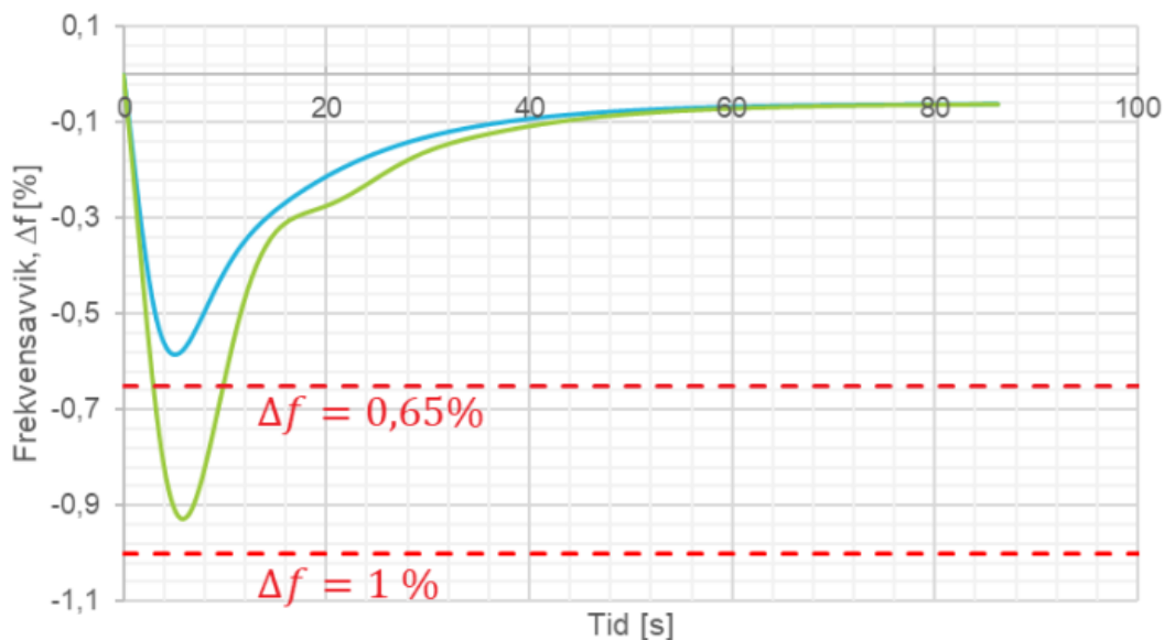
FIGUR 13-29: FREKVENSPRESPONS I TIDSPLANET VED 1% LASTPÅSLAG REFERERT P_{maks} . DE RØDE STIPLEDE LINJENE REPRESENTERER KRAVENE TIL MAKSIMALT TRANSIENT FREKVENSAVVIK. GRØNN (TYPE B OG C) OG BLÅ KURVER (TYPE D) ER EKSEMPLER PÅ FREKVENSFORLØP ETTER ET LASTSPRANG PÅ EGET OHMSK NETT.
