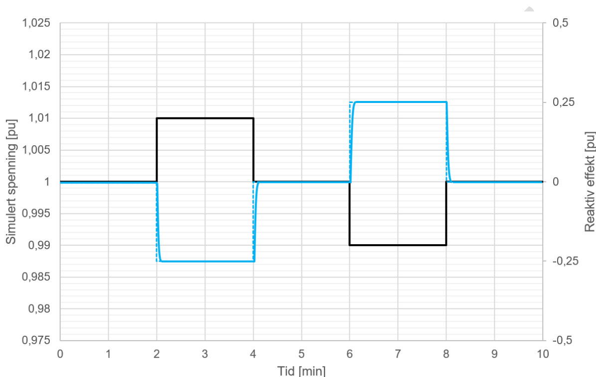
FIGUR 16-14: PRØVE VED STEG I SIMULERT NETTSPENNING.
