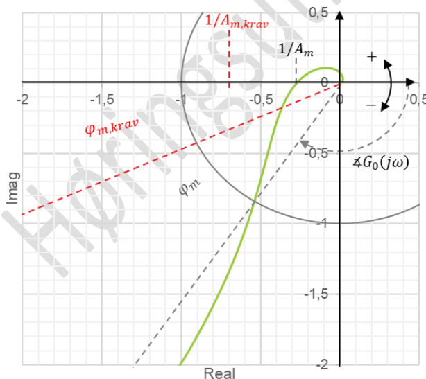
FIGUR 13-8: ILLUSTRASJON AV FREKVENSPANRESPONSEN (GRØNN) TIL G_0(s) , REF. LIGNING 13-1, I ET NYQUIST-DIAGRAM, HVILKET UTTRYKKER STABILITETEN TIL SYSTEMET. RØDSTIPLEDE LINJER INDIKERER KRAVENE TIL STABILITETSMARGIN. GRÅSTIPLEDE ER FAKTISK STABILITETSMARGIN.
