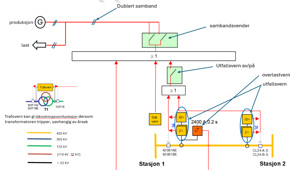
FIGUR 6-2 PRISIPPSKISSE FOR TILKNYTNINGSVERN VIST MED DUBLERT SAMBAND FOR TRANSMISJONSNETT
