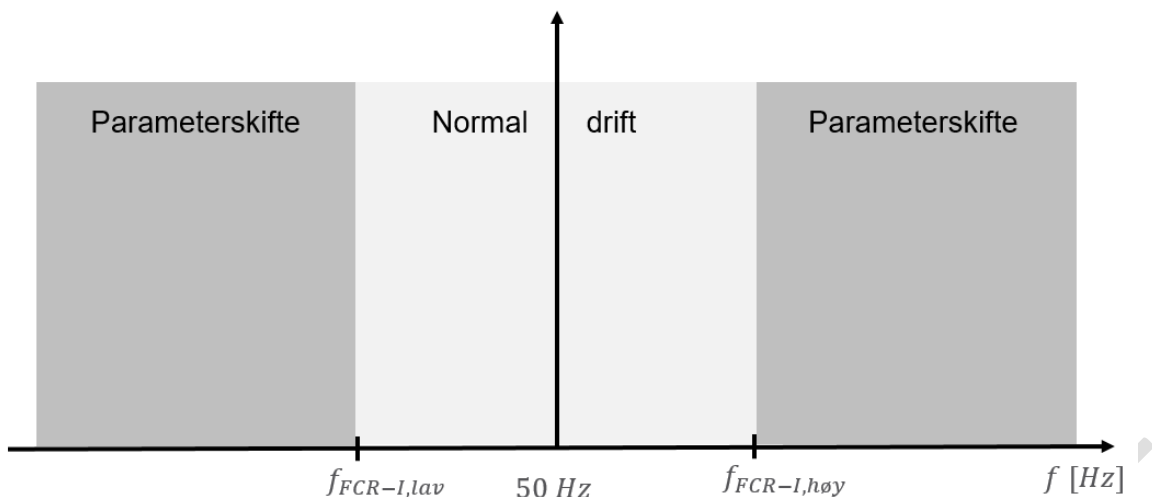
FIGUR 12-5: ILLUSTRASJON AV AUTOMATISK OG UFORSINKET AKTIVERING AV FCR VED KRITERIER FOR FCR-I.
