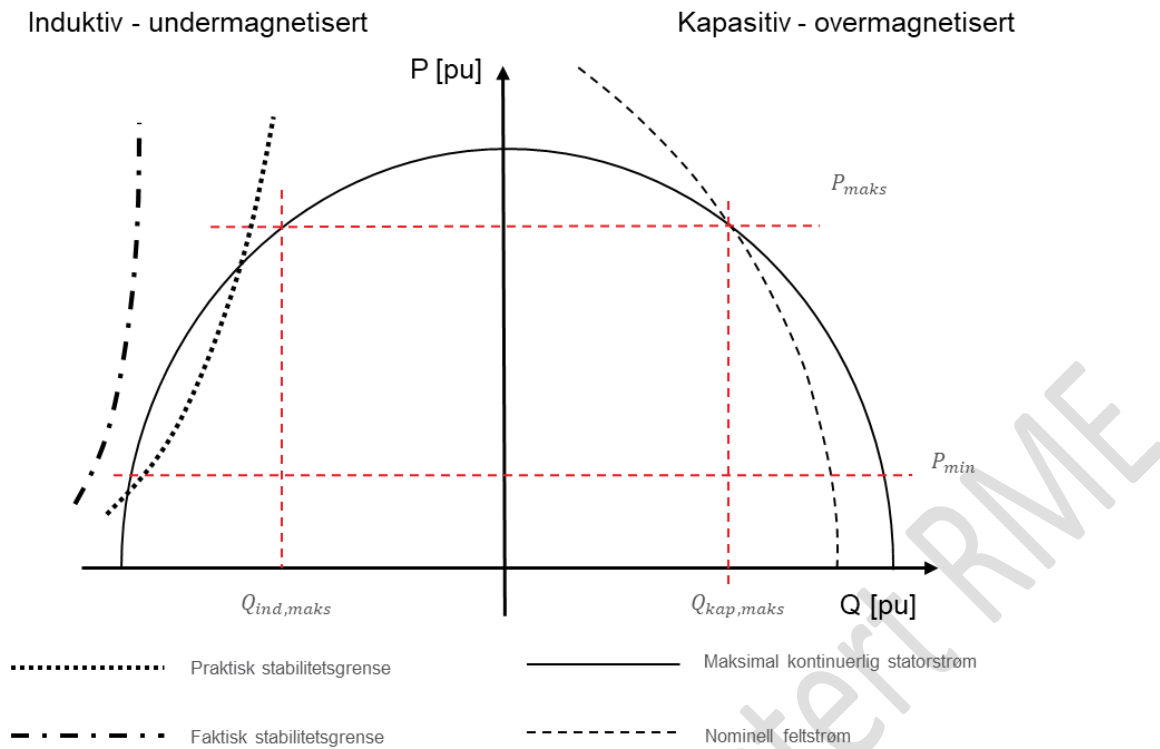
FIGUR 12-7: DRIFTSDIAGRAMMET TIL EN TYPISK SYNKROGENERATOR
