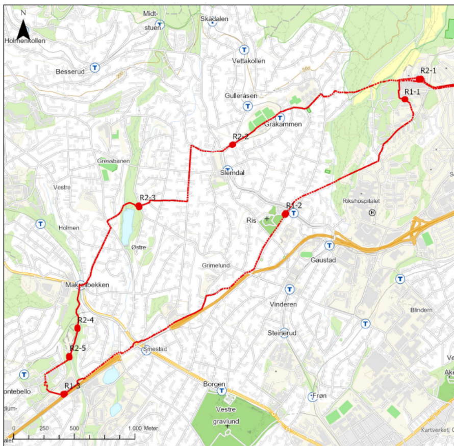
Figur 1. Oversikt over riggområdene langs kablene NV1 (sørligste) og NV2. Kablene er vist med rød siplert linje og riggområdene med røde prikker. Kilde: Statnetts riggplan, vedlegg 4.2..
