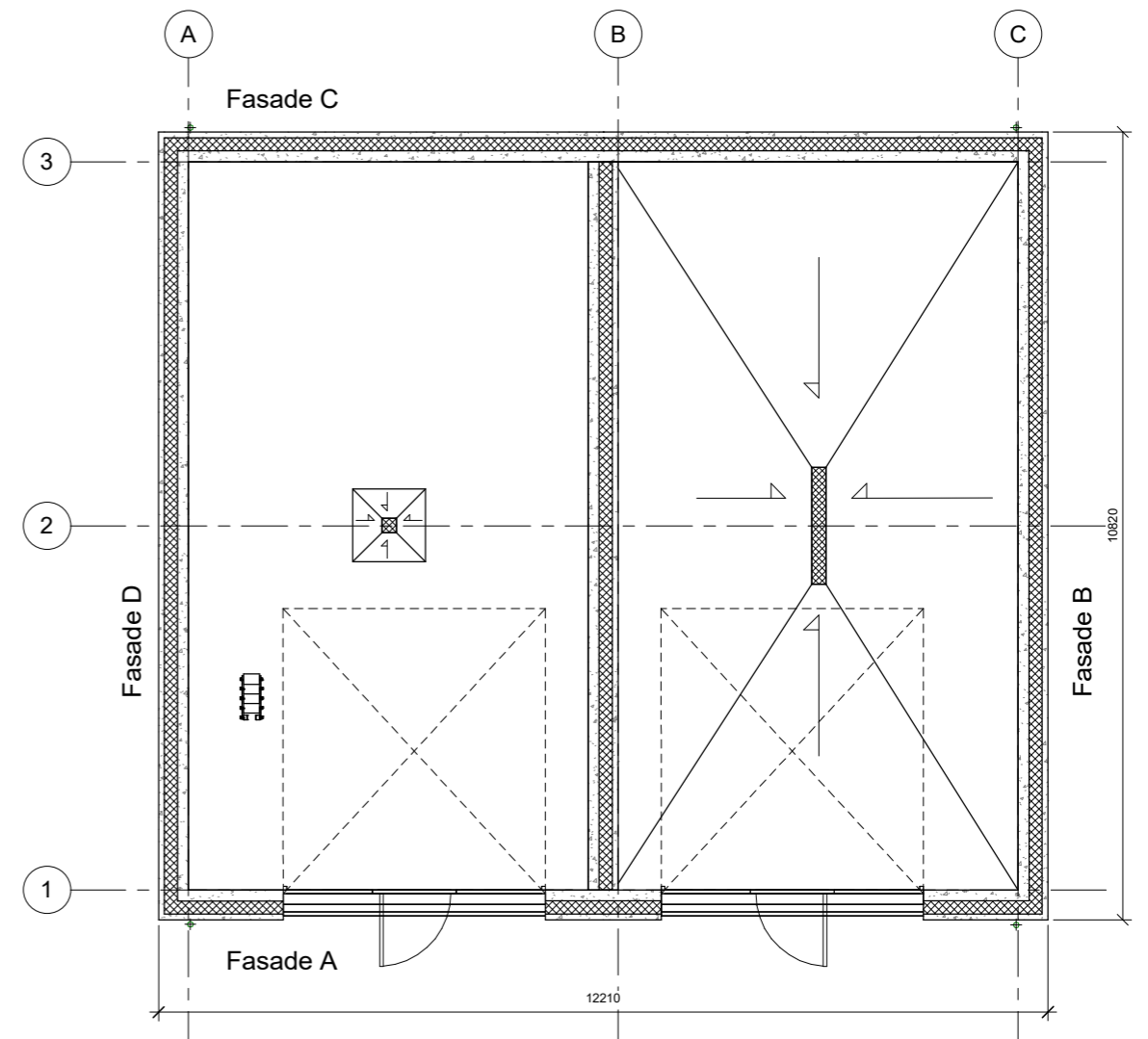
Plan 1. etasje 1 : 50
