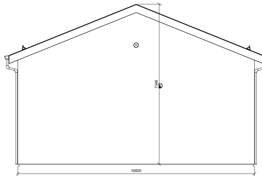
Fasade D 1 : 50
