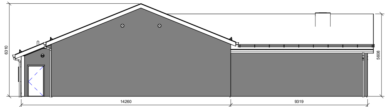
Fasade C 1 : 80
