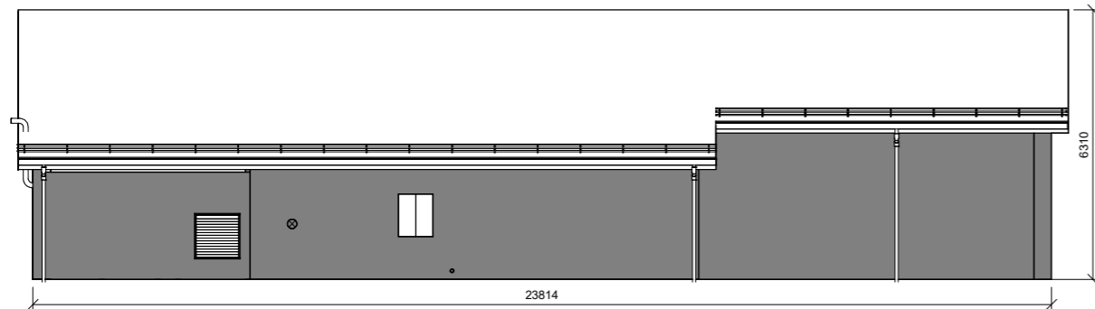
Fasade B 1 : 80
