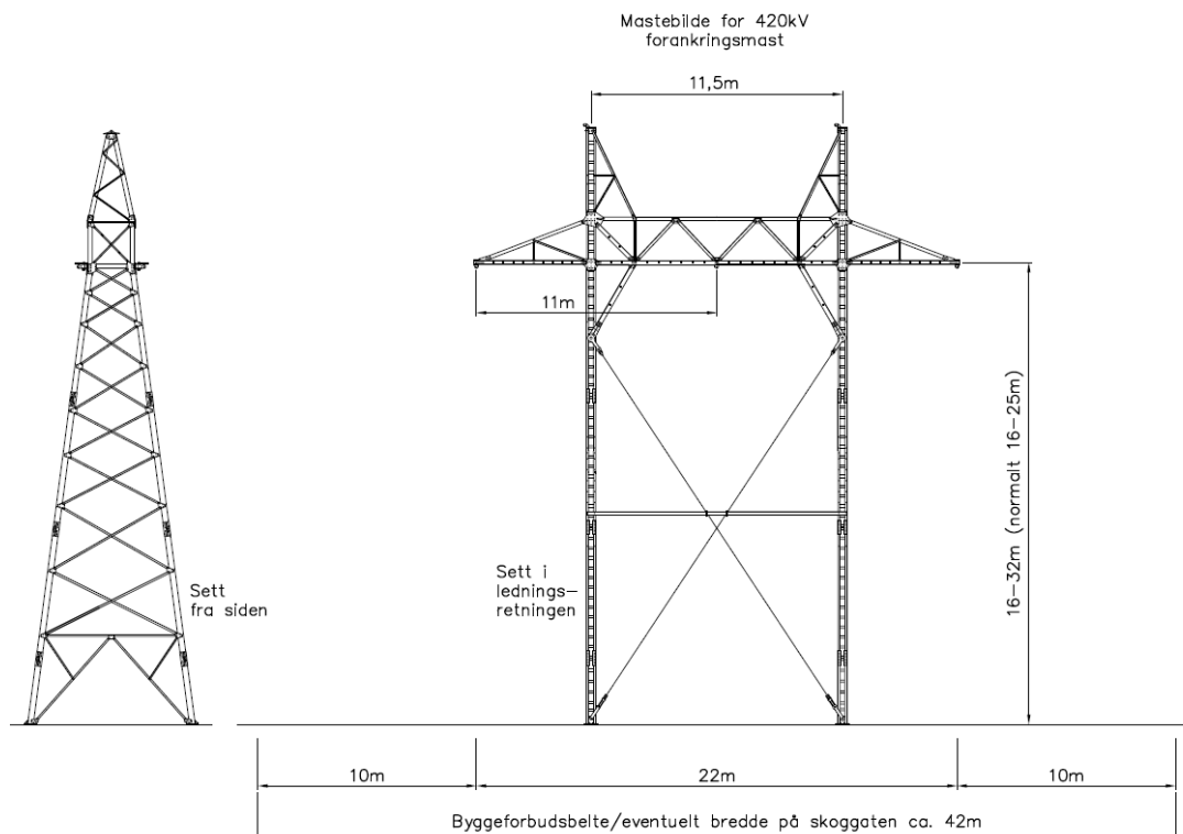
Figur 8 Illustrasjon av 420 kV forankringsmast
