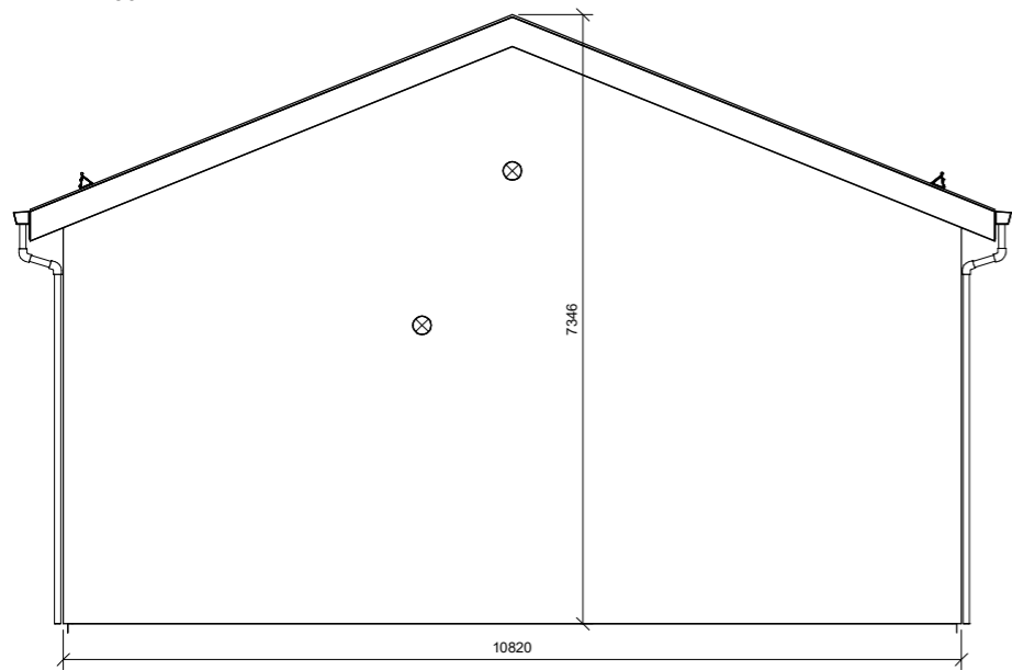
Fasade B 1 : 50
