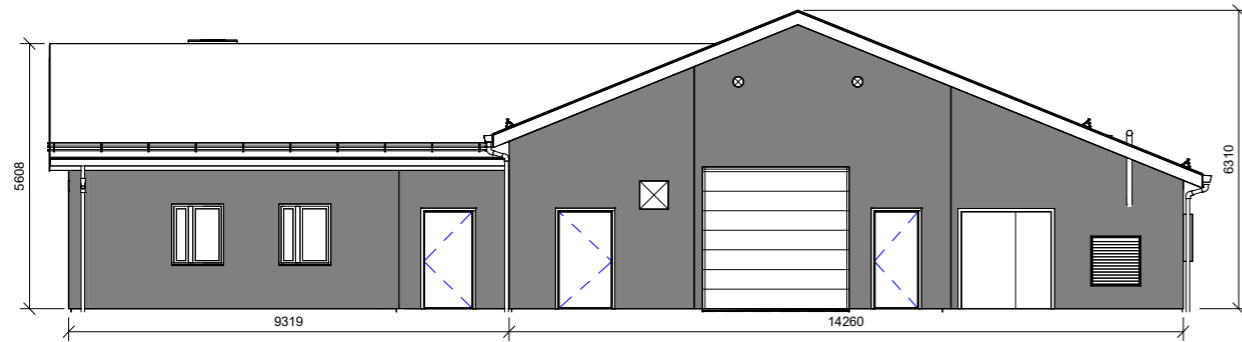
Fasade A 1 : 80
