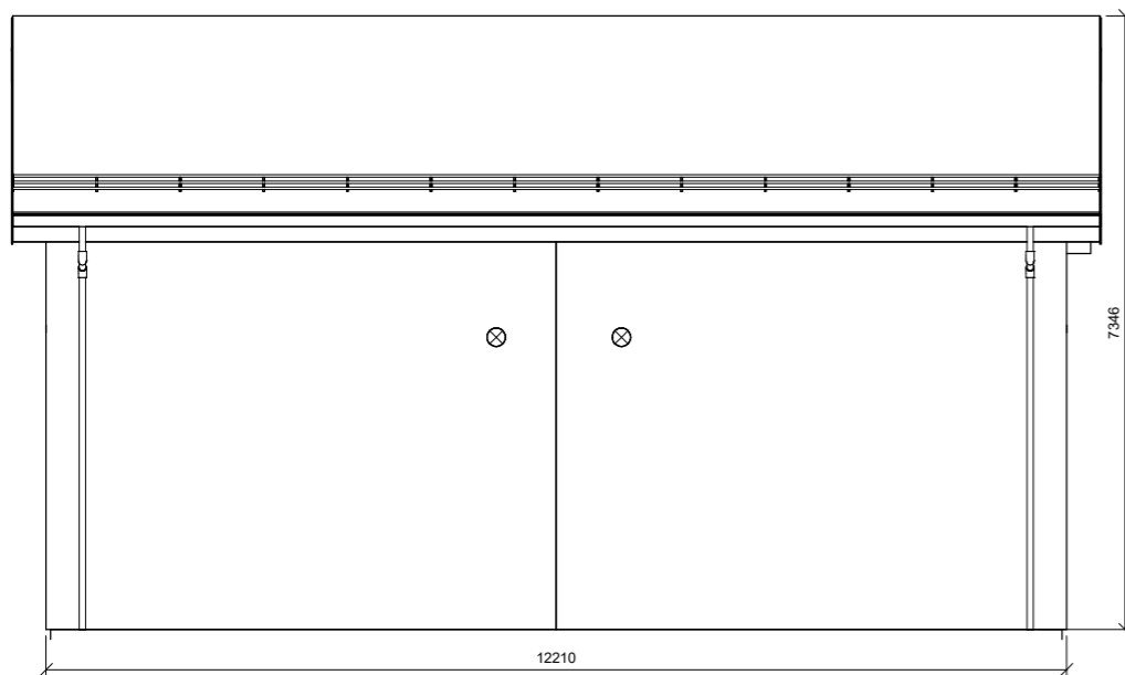
Fasade C 1 : 50
