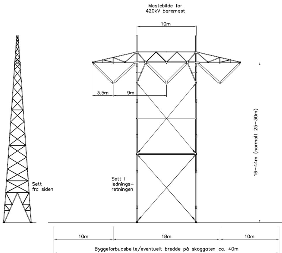
Figur 7 Illustrasjon av 420 kV bæremast
