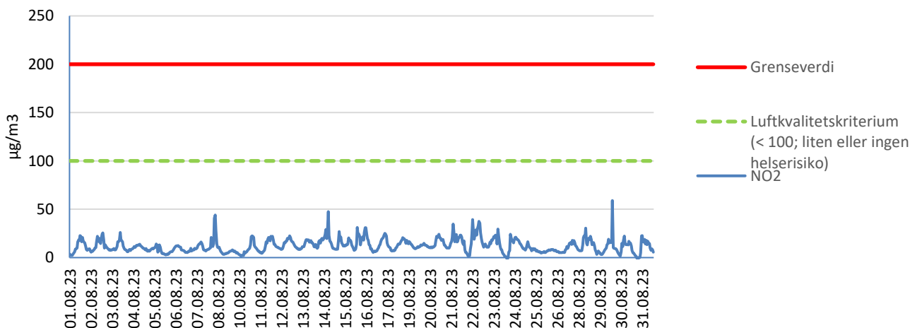
Figur 5.3. Timesmidler NO 2 ved Rektorhaugen i august.
