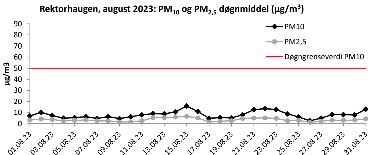
Figur 5.1. Døgnmidler \text{PM}_{10} og \text{PM}_{2,5} ved Rektorhaugen i august 2023, inkludert døgngrenseverdi for \text{PM}_{10} på 50 \mu\text{g}/\text{m}^3 .
