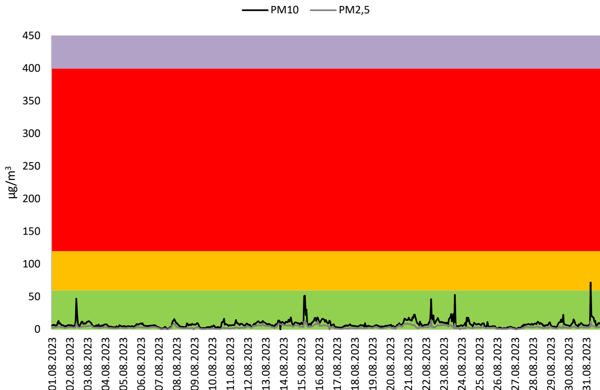
Figur 5.2. Timesmidler PM 10 og PM 2,5 ved Rektorhaugen i august 2023. Fargeklassifiseringen for varslingsklassene basert på helsevirkninger gjelder for PM 10 (svart linje). Grønn klasse: Liten eller ingen helserisiko, gul klasse: moderat helserisiko, rød klasse: betydelig helserisiko.
