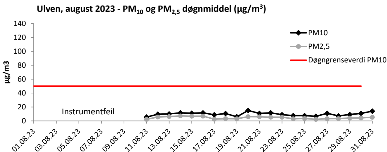
Figur 5.4 Døgn grenseverdier PM 10 og PM 2,5 ved Ulven i august. Data til og med 11. august kl. 13 mangler pga instrumentfeil.
