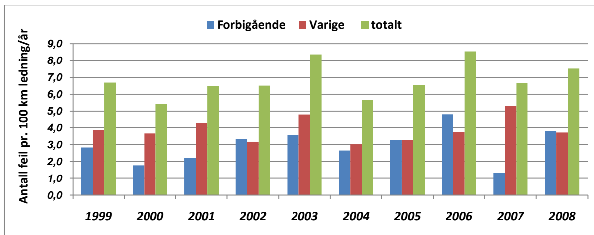
Figur 3.1 Feil på kraftledning som har ført til driftsforstyrrelser 1999-2008.
