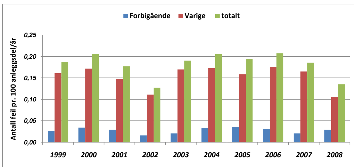
Figur 3.9 Feil på lastbrytere, skillebrytere og siklastbrytere som har ført til driftsforstyrrelser 1999-2008.
