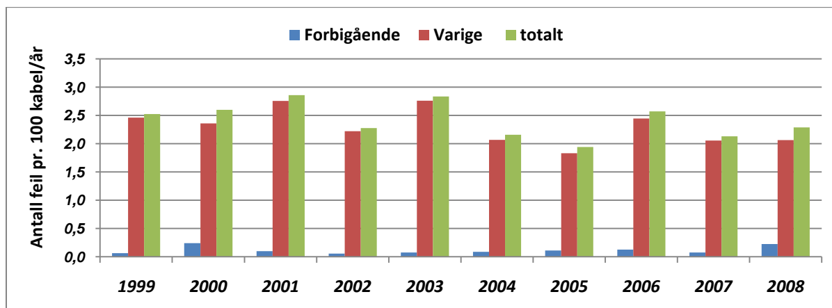
Figur 3.3 Feil på kabel som har ført til driftsforstyrrelser 1999-2008.
