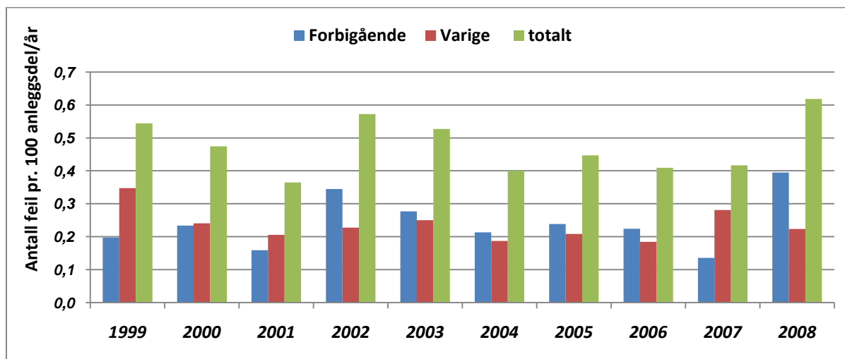
Figur 3.7 Feil på effektbryter som har ført til driftsforstyrrelser 1999-2008.
