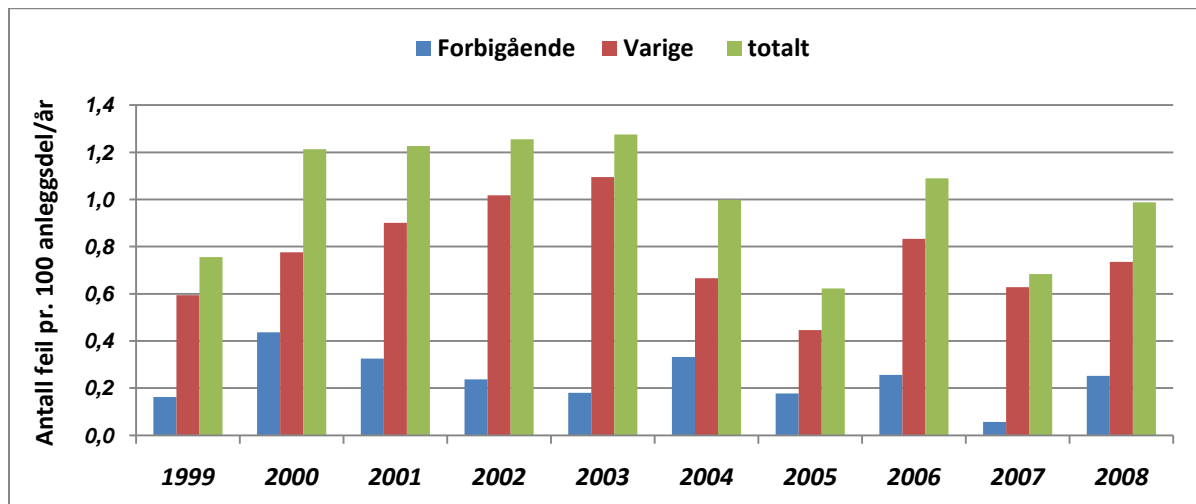
Figur 3.5 Feil på fordelingstransformator som har ført til driftsforstyrrelser 1999-2008.
