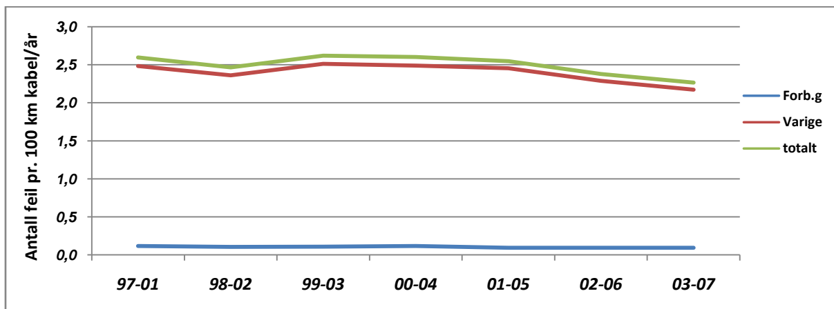
Figur 3.4 For å glatte ut årlige variasjoner, gi en mer riktig trend og en bedre tilpasning til Nordel statistikken, brukes her et glidende gjennomsnitt for de fem siste år.
