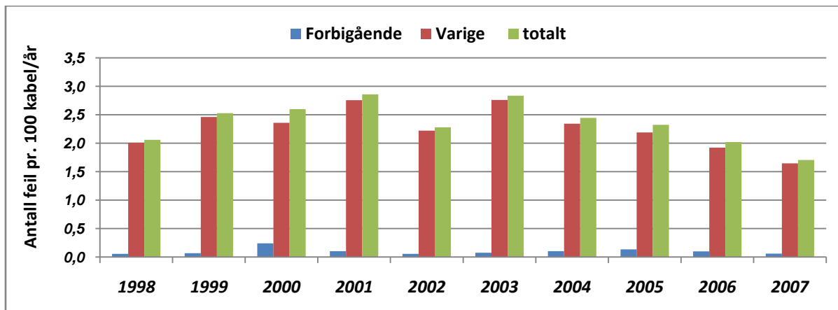
Figur 3.3 Feil på kabel som har ført til driftsforstyrrelser 1998-2007.
