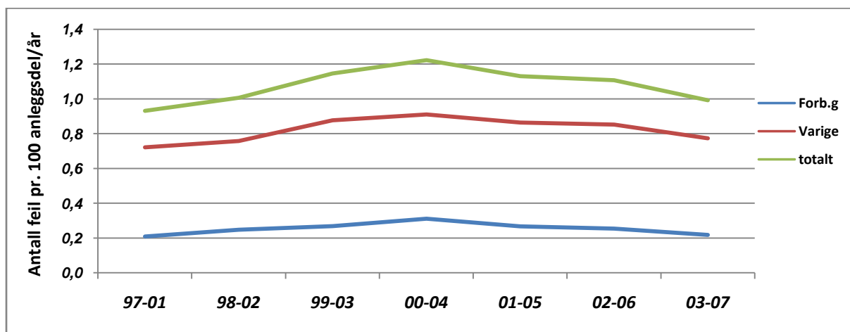
Figur 3.6 For å glatte ut årlige variasjoner, gi en mer riktig trend og en bedre tilpasning til Nordel statistikken, brukes her et glidende gjennomsnitt for de fem siste år.
