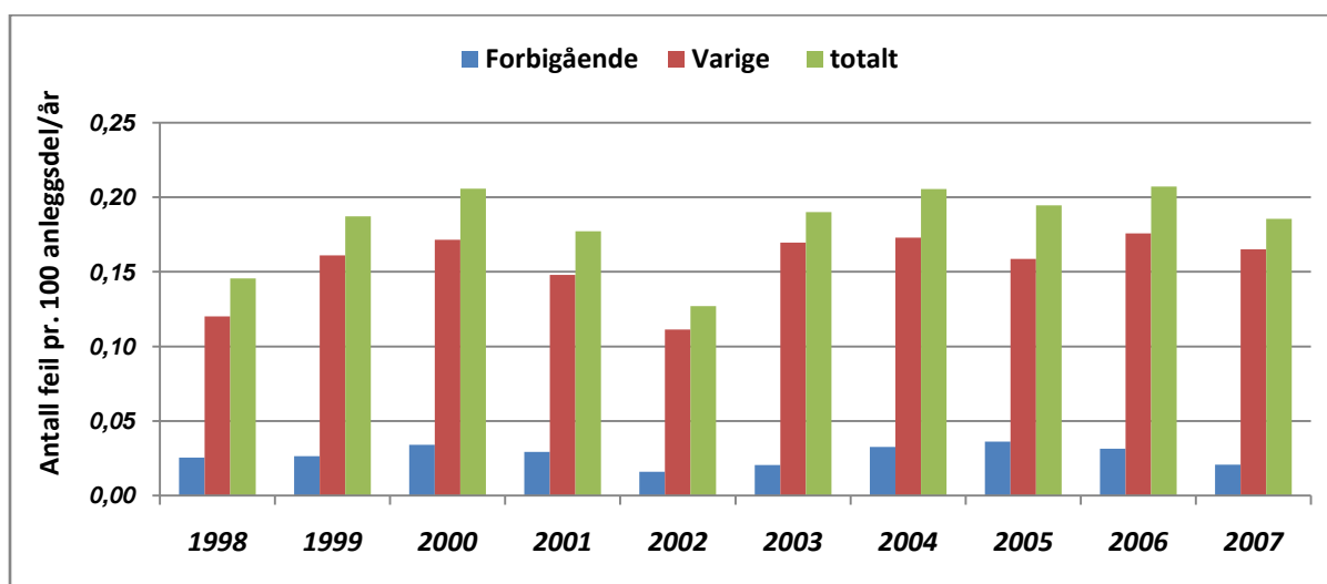
Figur 3.9 Feil på lastbrytere, skillebrytere og siklastbrytere som har ført til driftsforstyrrelser 1998-2007.
