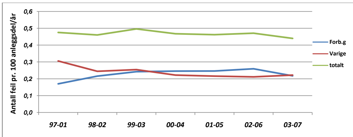
Figur 3.8 For å glatte ut årlige variasjoner, gi en mer riktig trend og en bedre tilpasning til Nordel statistikken, brukes her et glidende gjennomsnitt for de fem siste år.
