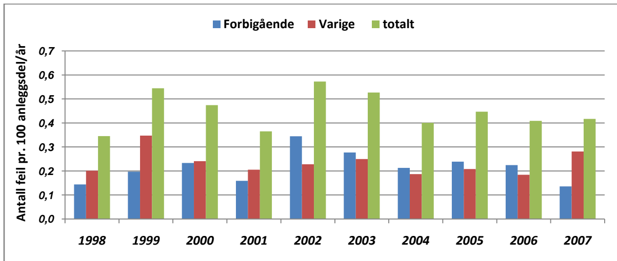
Figur 3.7 Feil på effektbryter som har ført til driftsforstyrrelser 1998-2007.
