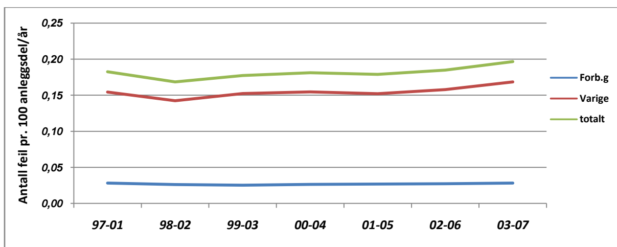
Figur 3.10 For å glatte ut årlige variasjoner, gi en mer riktig trend og en bedre tilpasning til Nordel statistikken, brukes her et glidende gjennomsnitt for de fem siste år.
