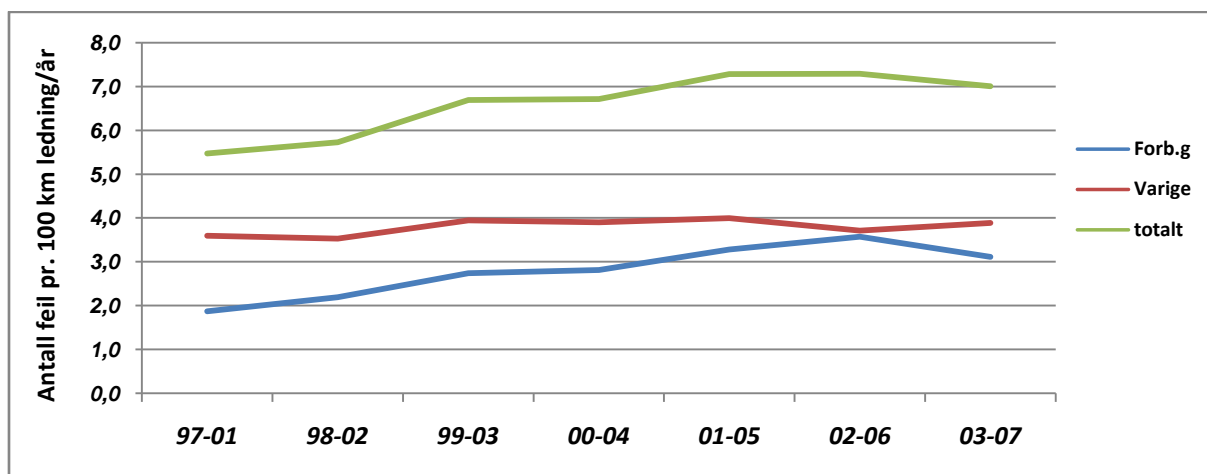
Figur 3.2 For å glatte ut årlige variasjoner, gi en mer riktig trend og en bedre tilpasning til Nordel statistikken, brukes her et glidende gjennomsnitt for de fem siste år.
