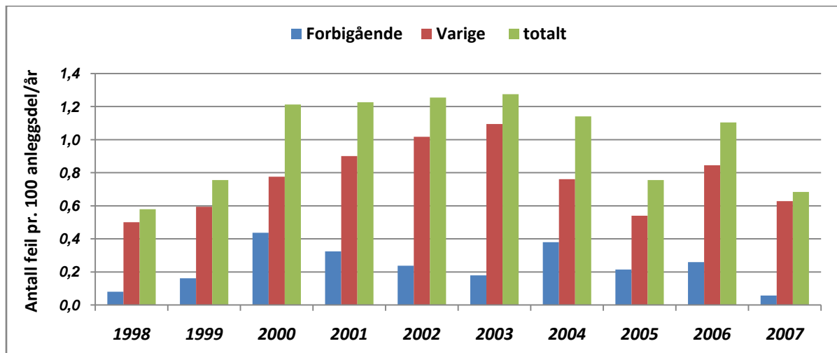
Figur 3.5 Feil på fordelingstransformator som har ført til driftsforstyrrelser 1998-2007.
