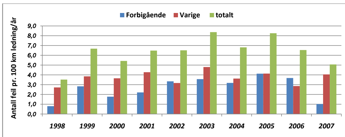
Figur 3.1 Feil på kraftledning som har ført til driftsforstyrrelser 1998-2007.
