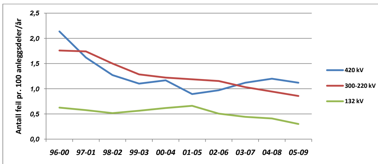
Figur 3.8 For å glatte ut årlige variasjoner, gi en mer riktig trend og en bedre tilpasning til Entso-E Nordic statistikken, brukes her et glidende gjennomsnitt for de fem siste år.
