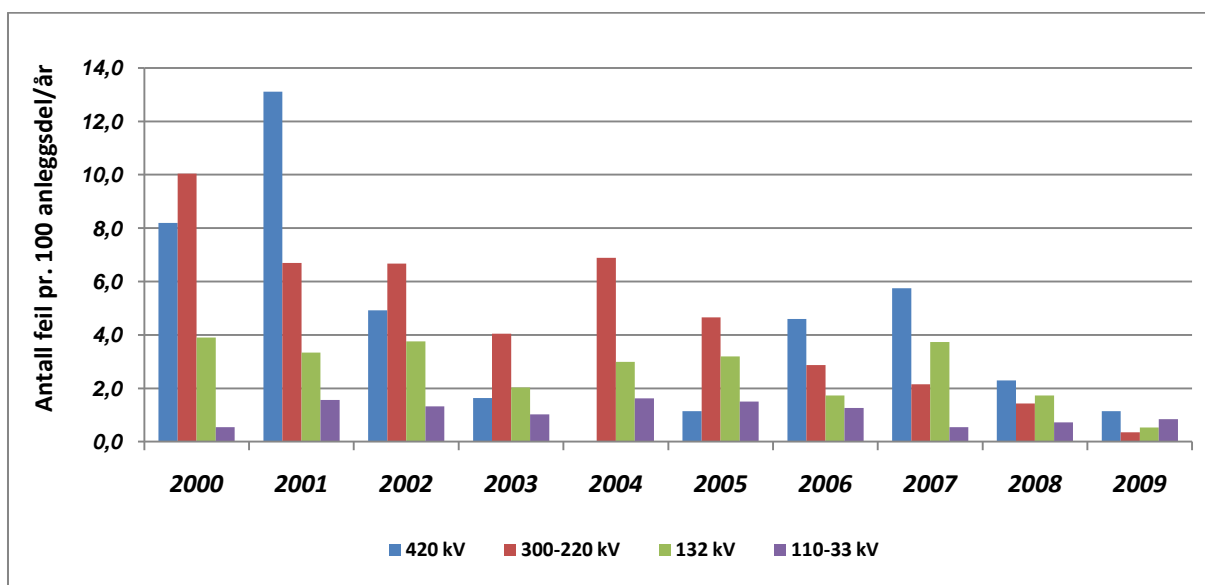
Figur 3.11 Feil på vern og kontrollutstyr for anleggsdel krafttransformatorer fordelt på år og spenningsnivå.
