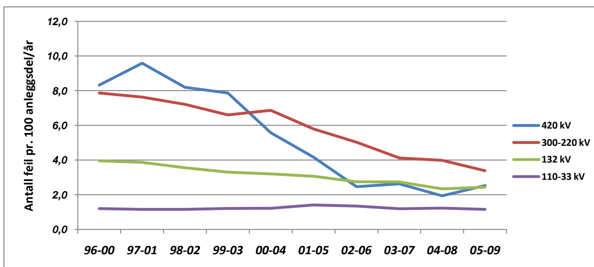
Figur 3.12 For å glatte ut årlige variasjoner, gi en mer riktig trend og en bedre tilpasning til Entso-E Nordic statistikken, brukes her et glidende gjennomsnitt for de fem siste år.
