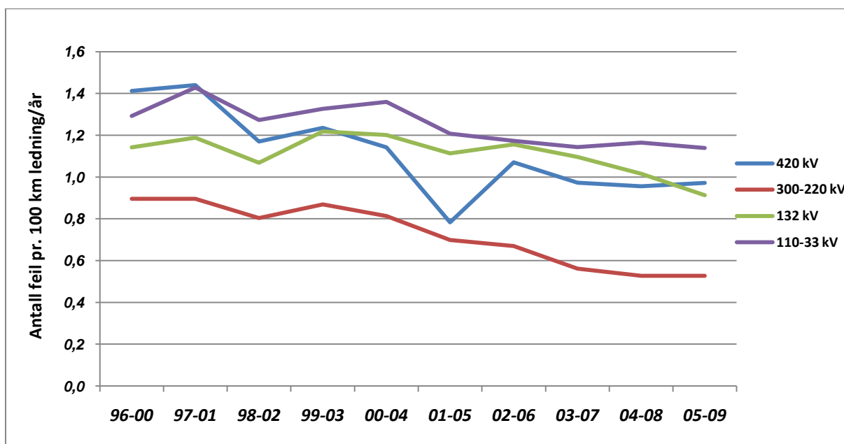
Figur 3.2 For å glatte ut årlige variasjoner, gi en mer riktig trend og en bedre tilpasning til Entso-E Nordic statistikken, brukes her et glidende gjennomsnitt for de fem siste år.
